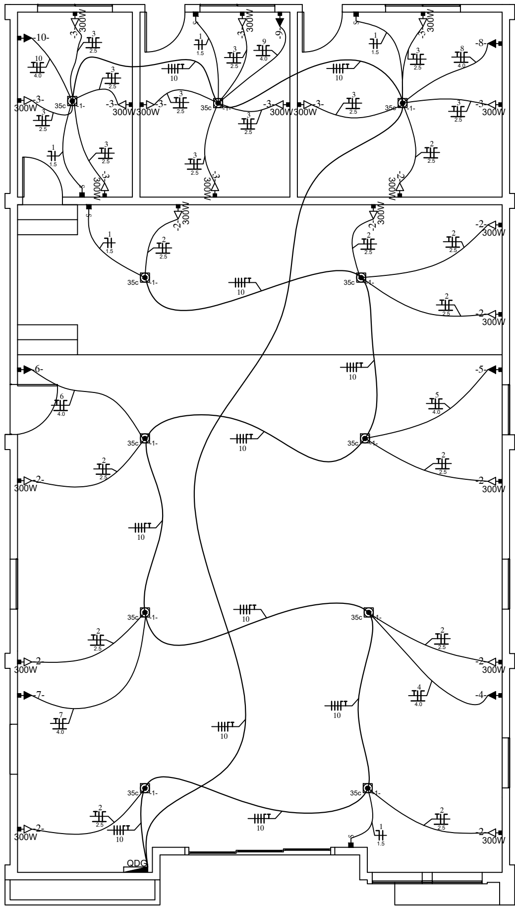
PLANTA INST. ELÉTRICA ESCALA: 1:75
